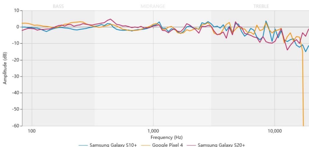
Bild 16: Frequenzgang von Samsung-Geräten 4 der für die Aufnahme verwendeten Gerätegeneration
