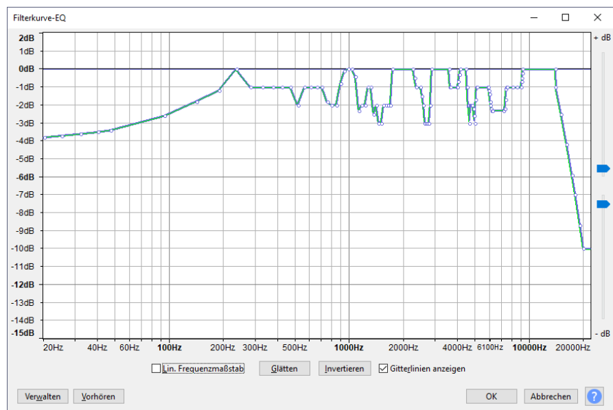
Bild 17: Realer Frequenzgang Stereo-Mikrofon Tascam DR05X / SN 2052166 mit Tascam Windmuff WS-11
