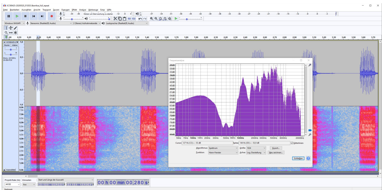
Bild 11: Spektrogramm Wachtelkönig-Ruf für ein Zeitfenster von 36ms
