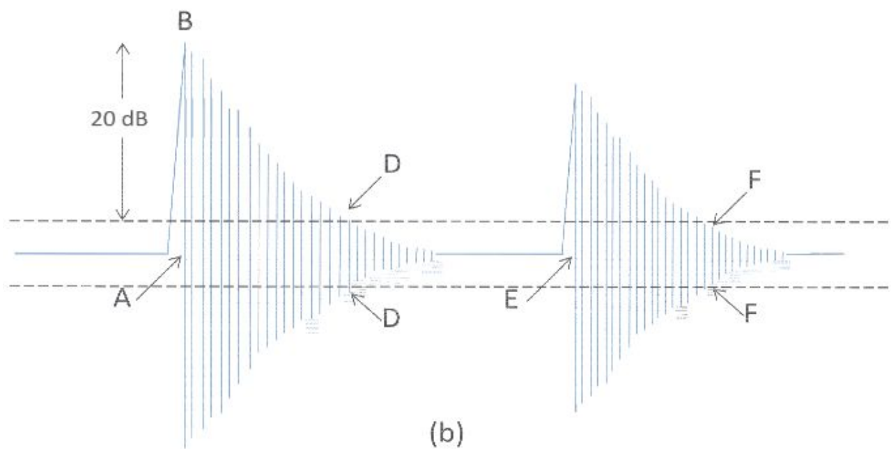
Bild 13: Bildzitat (Abb. 5, Seite 17) aus [Klein]: Idealisierte Wellenform von Impulslärm nach Pfander
